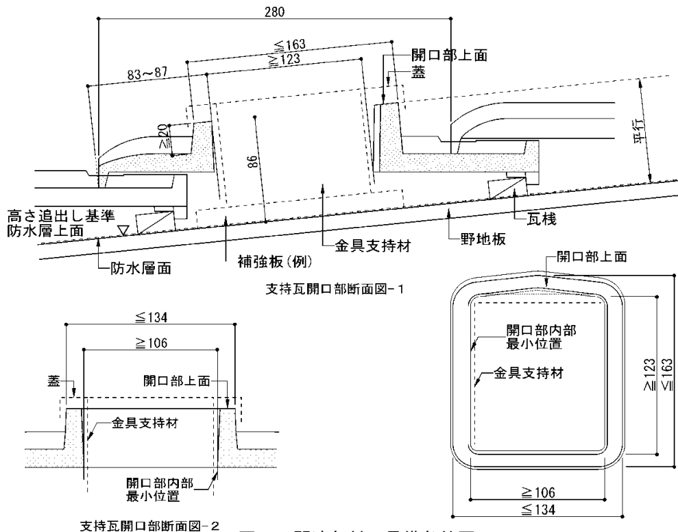
図2－関連部材の具備条件図 支持瓦開口部断面図
