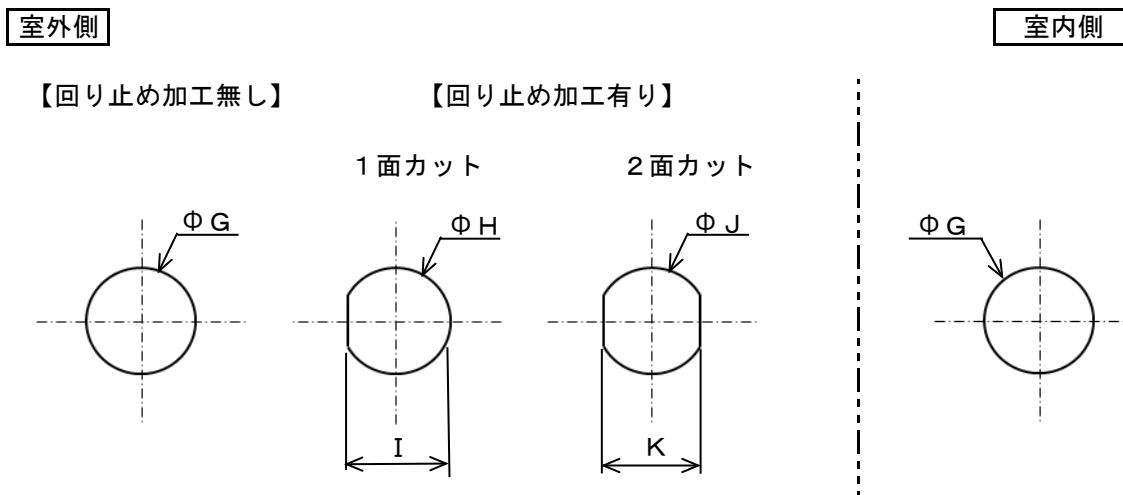
図2－取付穴の加工形状
