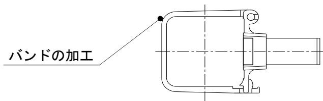
図2ーバンドの加工の例
