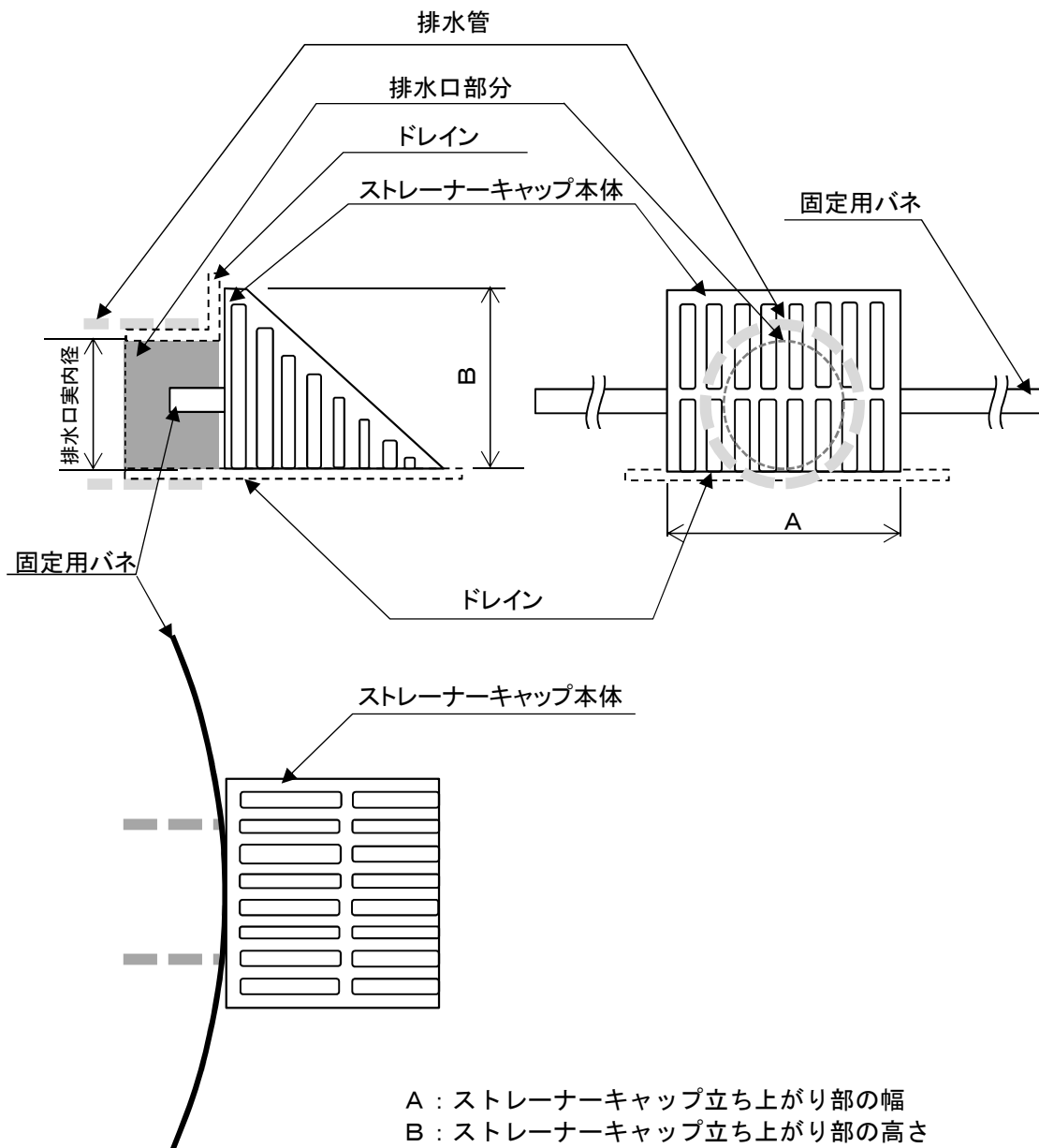
図1 - 標準(共通)化の部位
