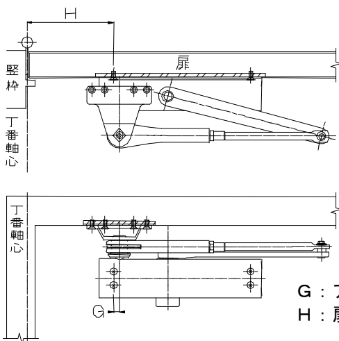
図2－推奨寸法の部位
