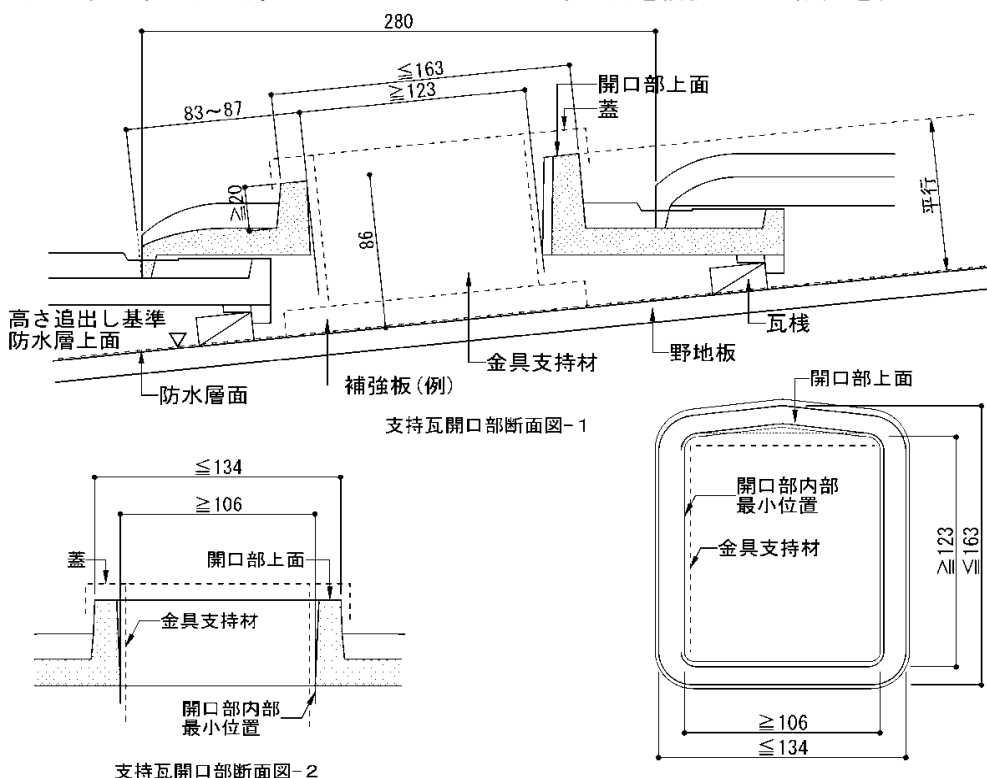
図 2－関連部材の具備条件図
