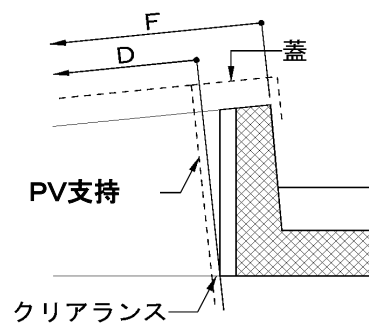
図5 - c - c 断面図
