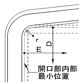
図7 - 開口部水上部コーナー平面図
