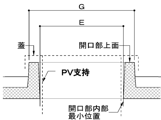
図4 - b - b 断面図
