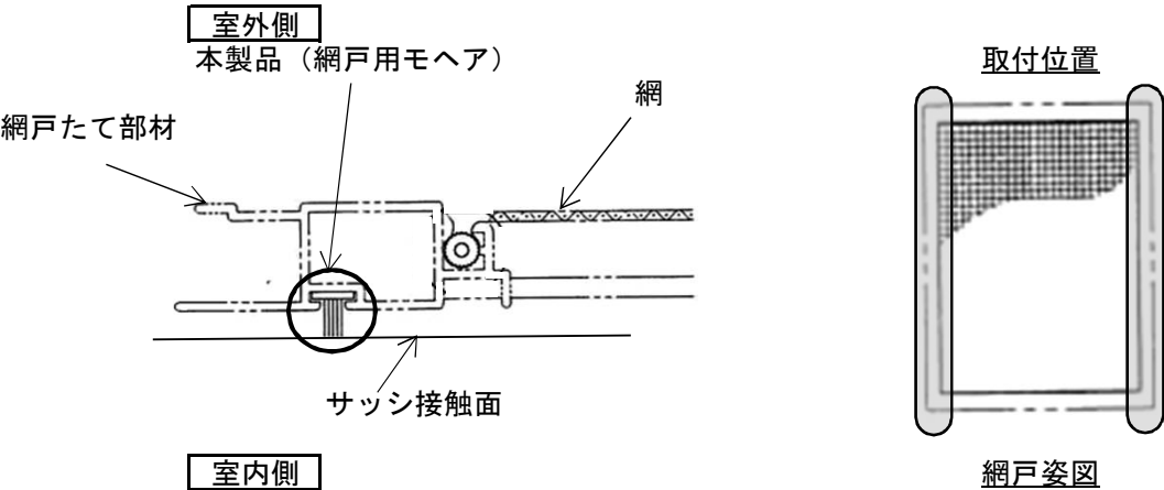
図 2－納まり図
