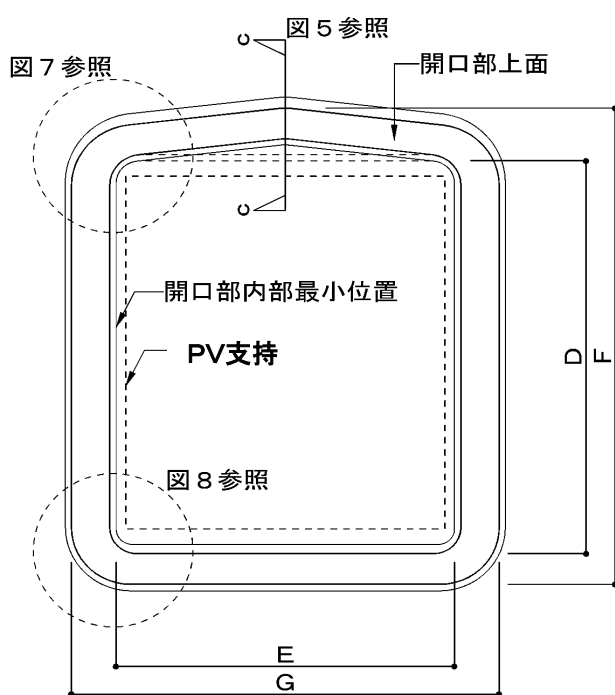
図6 - P V 支持材設置用開口部平面図
