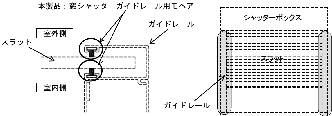
図2ー本製品の納まり図
